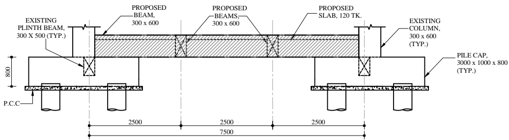
SECTION - A-A (SCALE - 1 : 50)
